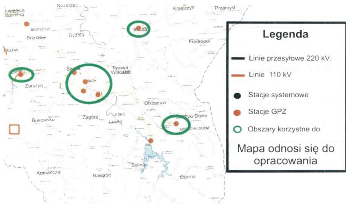
Mapa 6. Sieć elektroenergetyczna 110kV na terenie gminy i obszarach powiązanych
